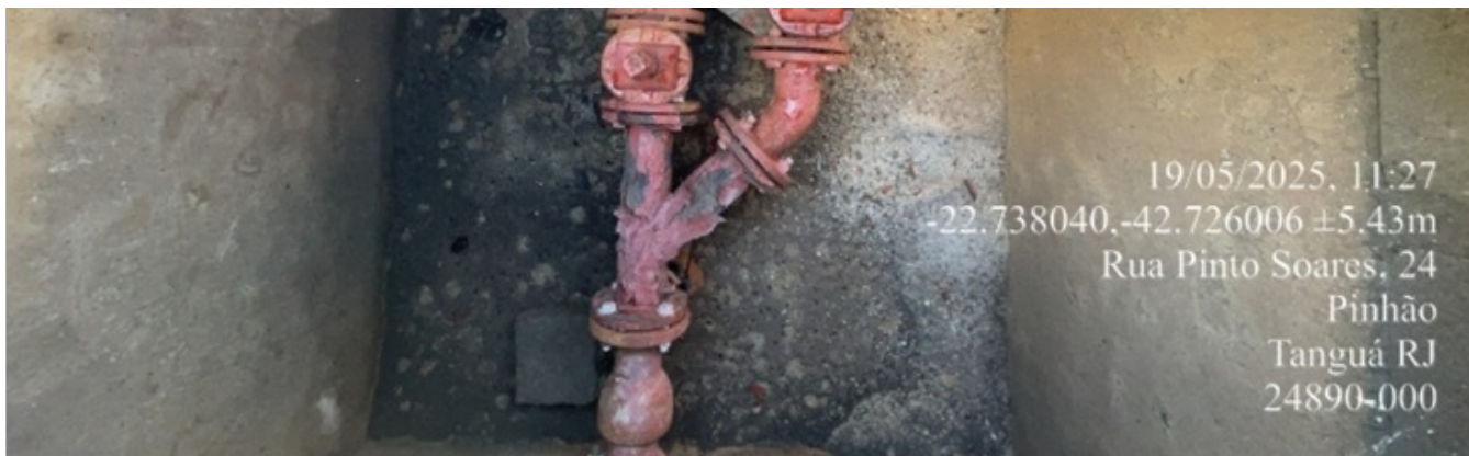
Foto 7 – Tubulação de recalque, válvulas de retenção e fechamento.
