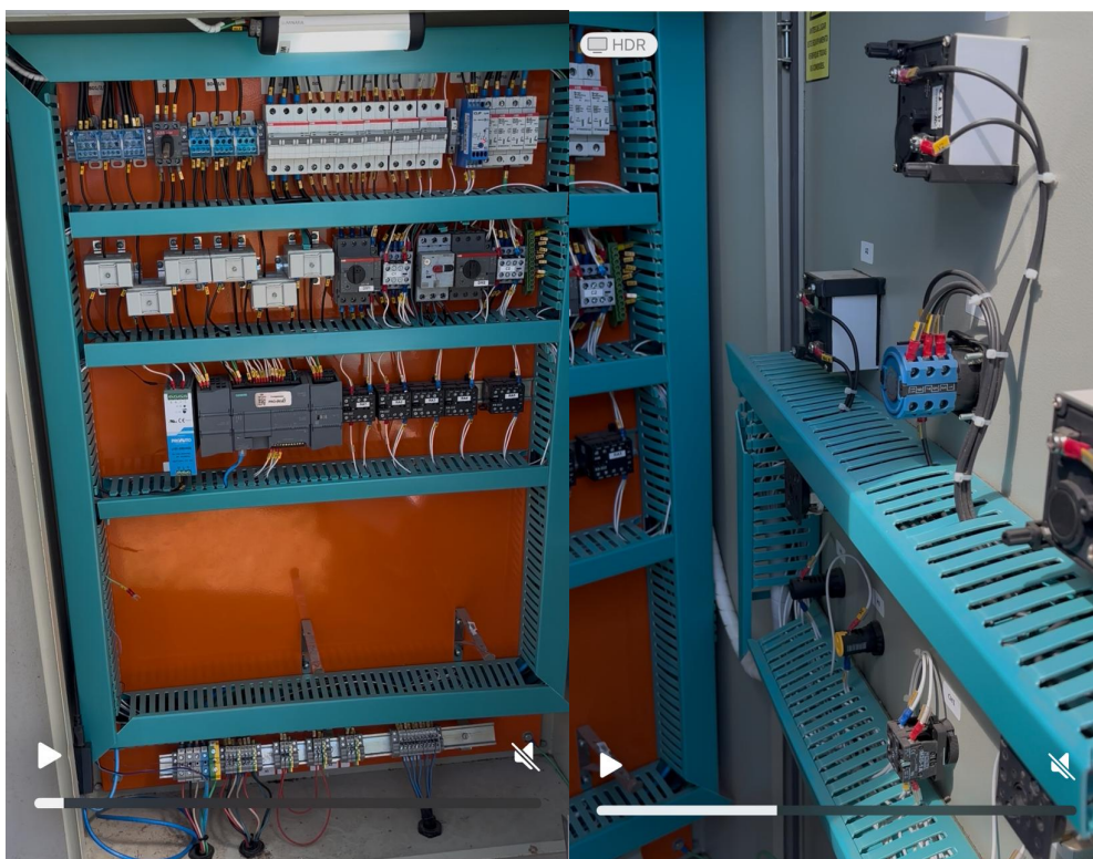
Fotos 4 – Quadro elétrico com telemetria
