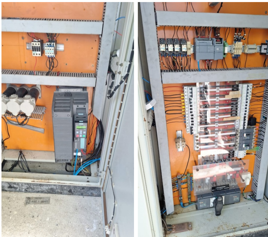
Fotos 3 e 4— Quadros elétricos com telemetria, proteção e inversor de frequência
