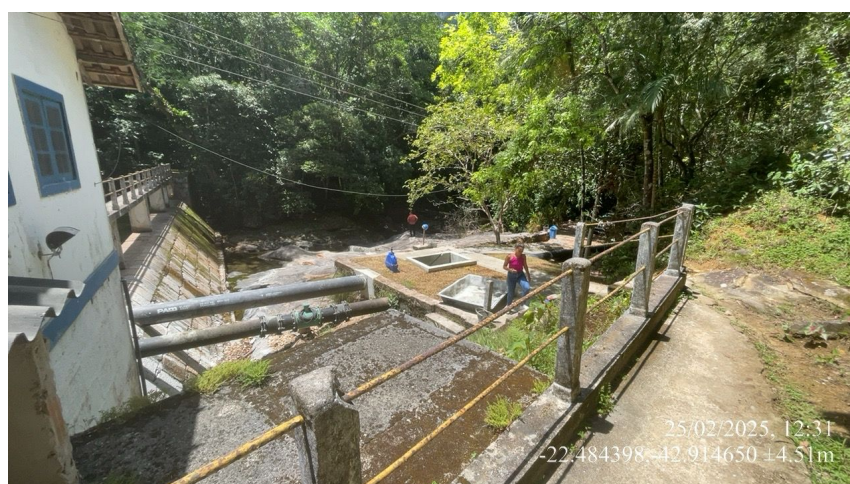
Foto 5 – Vista geral da barragem e tubulação
