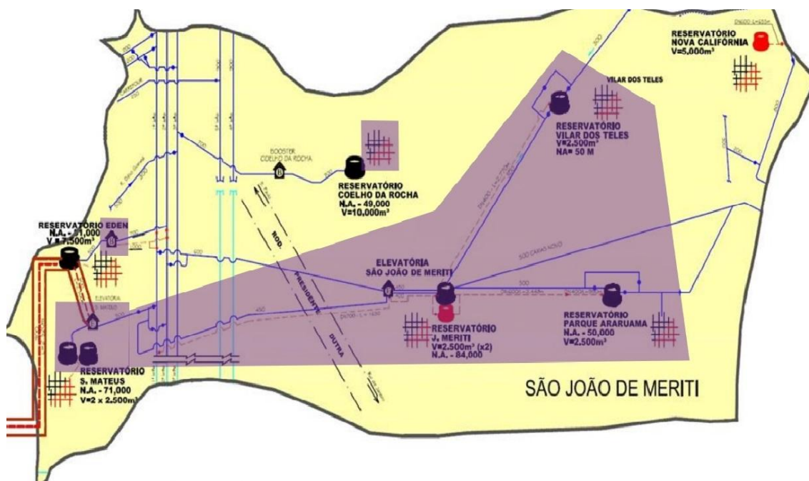
ESQUEMA DO SISTEMA DE SÃO JOÃO DE MERITI
