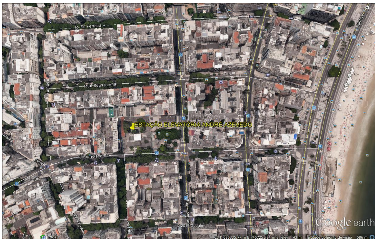
LOCALIZAÇÃO DA ESTAÇÃO ELEVATÓRIA DE ESGOTO ANDRÉ AZEVEDO - COPACABANA
