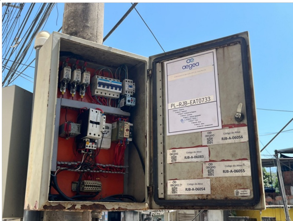
Foto 6 – Painel de automação enferrujado sem sinalização de risco de choque elétrico
