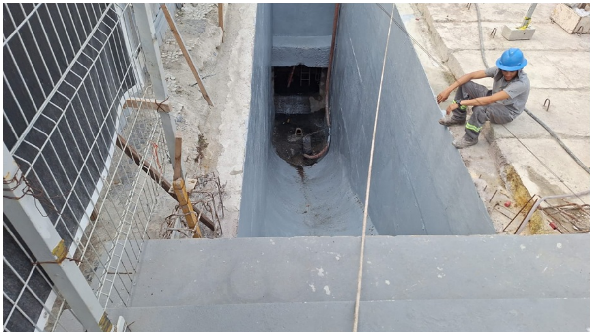
Fotos 7 – Reparo da base do acoplamento do parafuso; Vista da impermeabilização do poço após a concretagem, com drenagem do esgoto vazado pelas comportas, através de bomba sapo .
