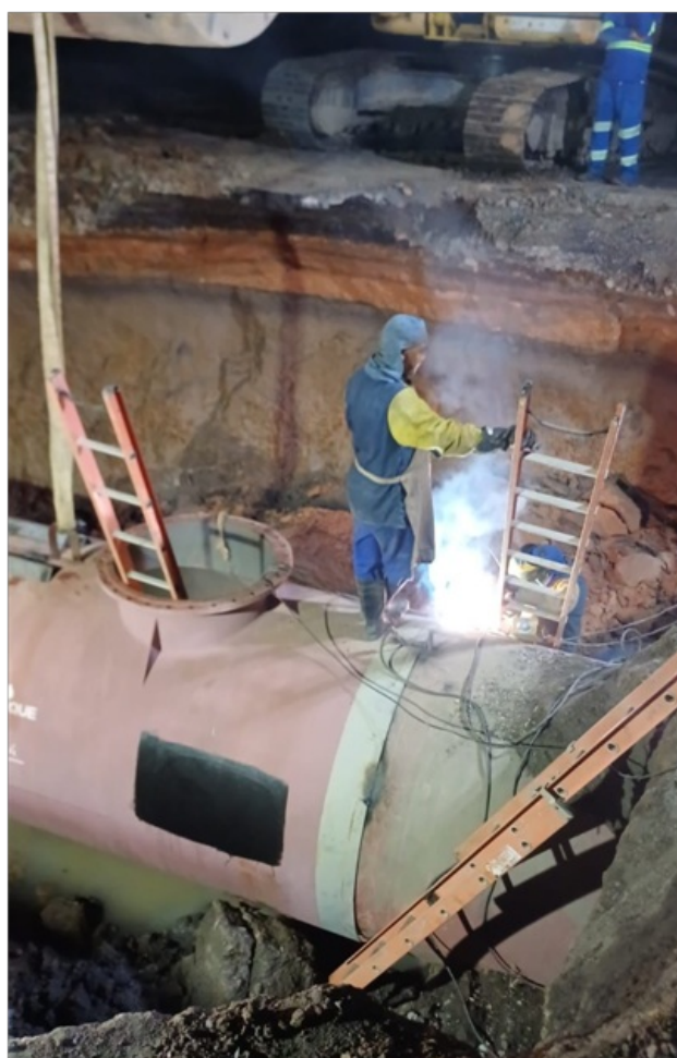
Foto 6 - Trabalhos de soldagem sendo realizados
