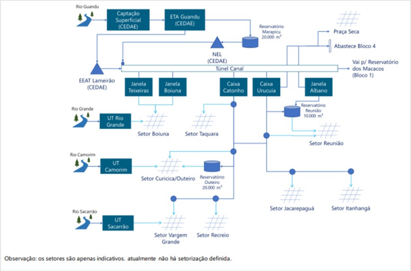
Figura 1 – Diagrama de Blocos: SAA Rio de Janeiro / Bloco2 (Fonte: Relatório de Diagnóstico dos Sistemas Operacionais Bloco 2. Em 22 de abril de 2022)
