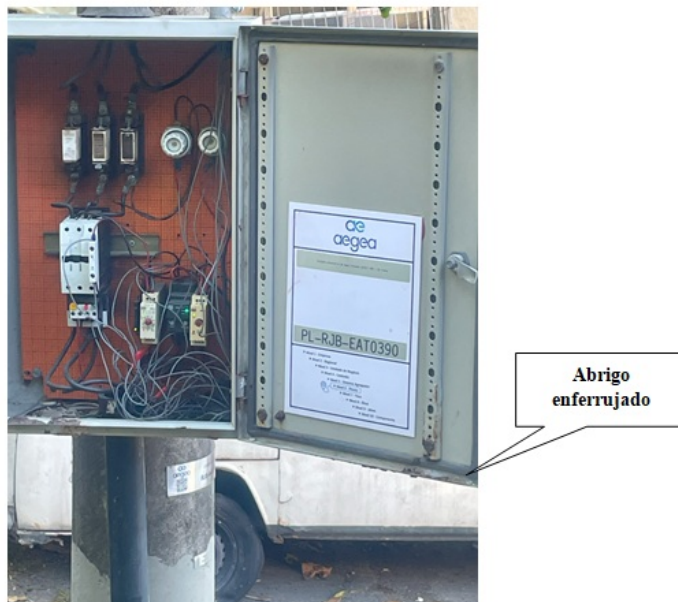
Figura 3 - Abrigo do painel de controle enferrujado e aberto
