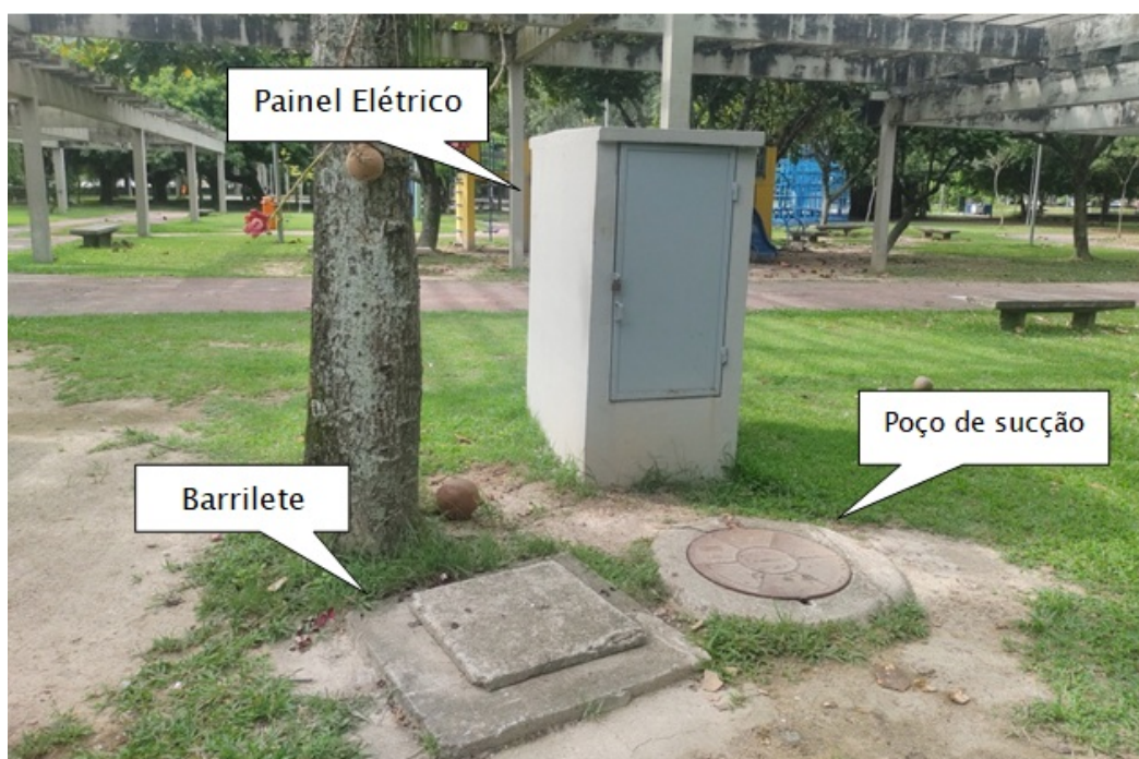
Foto 1 - EEE Parque dos Patins e identificação dos seus elementos.
