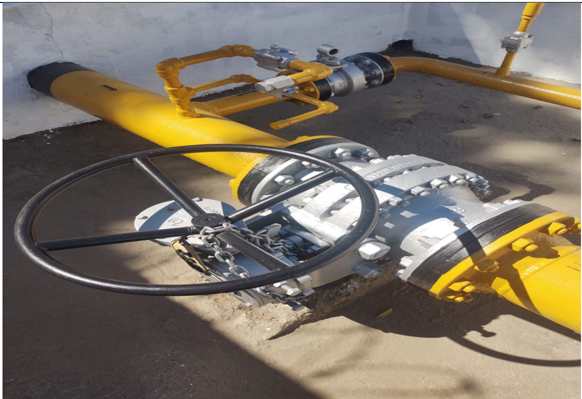
Foto 2: Válvula de linha e duto de aço 8".
