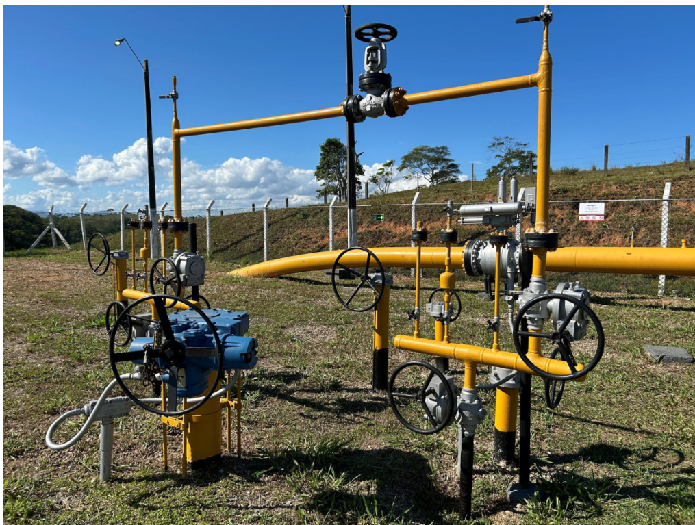
Foto 4: Válvulas de bloqueio e manobra para o canhão lançador de PIG (ao fundo).
