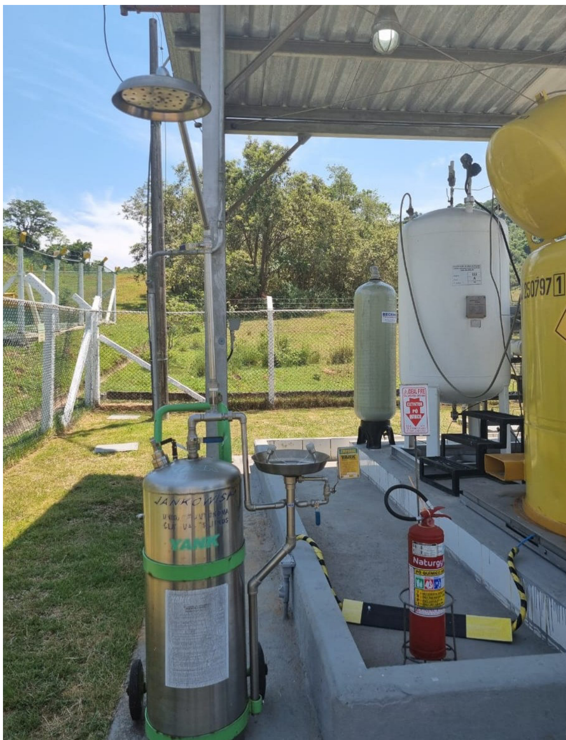
Foto 11: Extintor, lava olhos e chuveiro da estação de medição.
