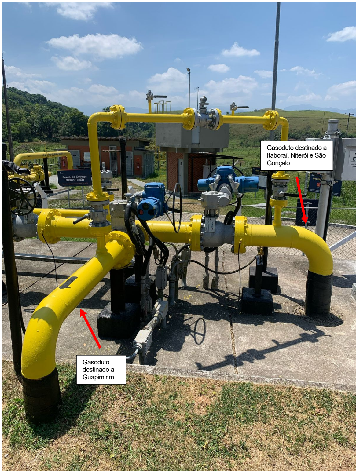
Foto 7: Redistribuição da tubulação com ramificações para Itaboraí e Guapimirim.
