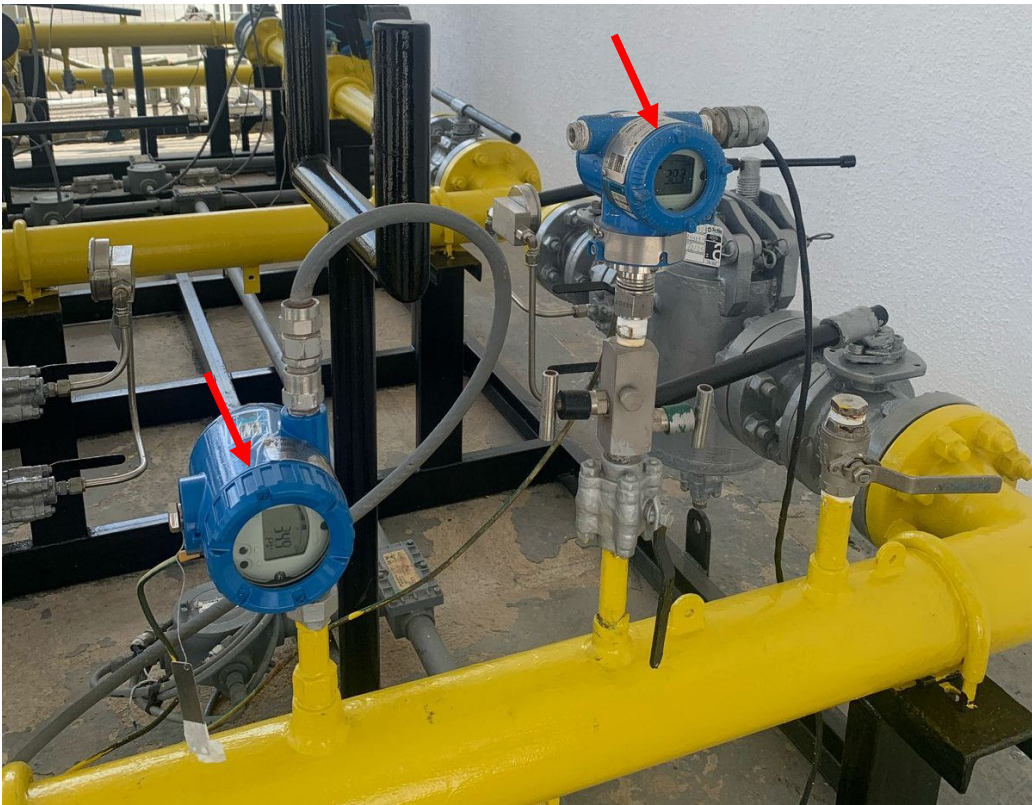
Foto 4: Medidores de temperatura e de pressão, respectivamente, no sistema de filtragem e medição.
