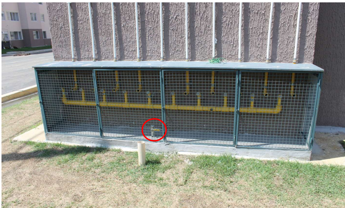
Foto 3 : Ponto de entrega de gás para alimentação dos medidores
