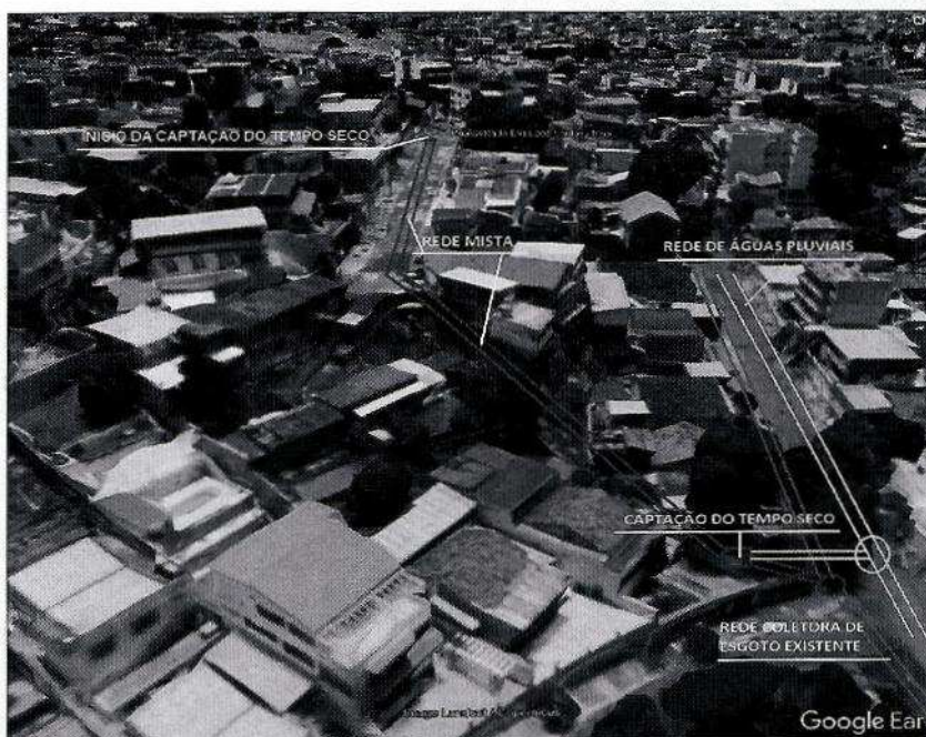
Esquema - Captação de Tempo Seco (fig 09)
